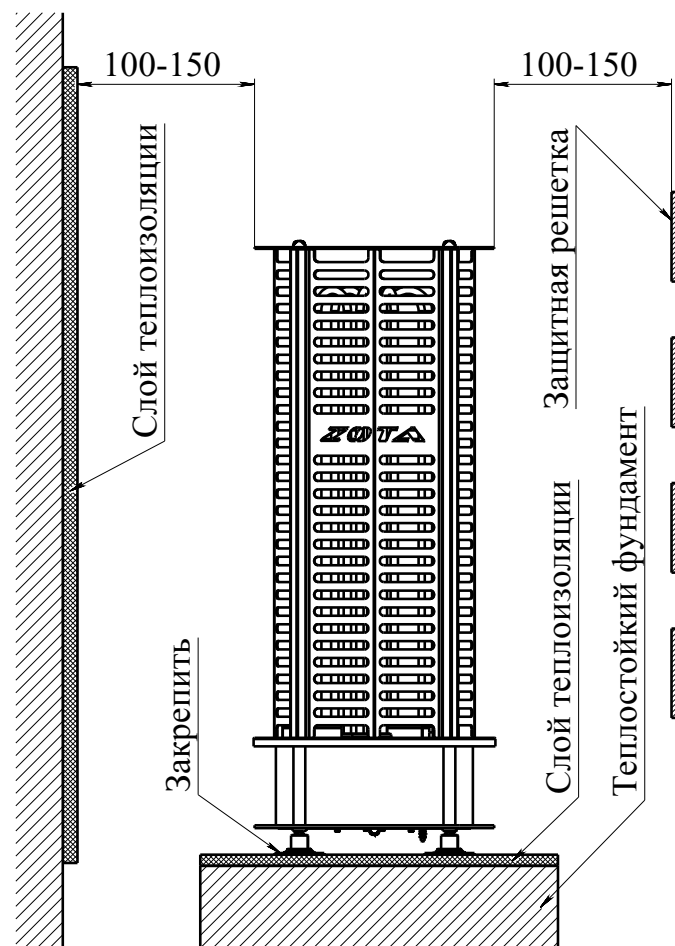
Рис.2 Установка электрокаменки
