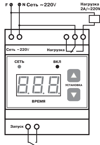
Рис.2 Схема подключения реле времени
