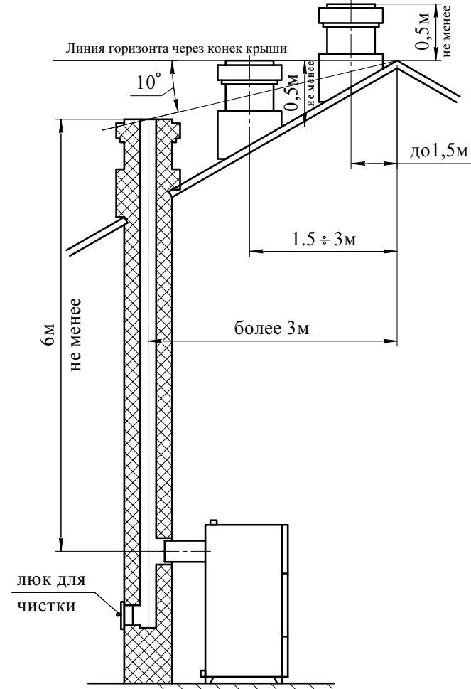
Рис. 7 Варианты установки дымовой трубы
