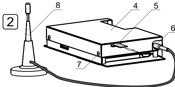
Рис.1 Конструкция и подключение модуля GSM
