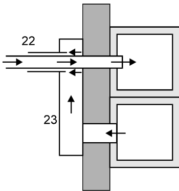
Двухходовая дымовая труба
