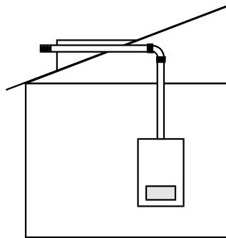
Горизонтальная дымовая труба (с воздухопроводом и дымоходом "труба в трубе") ввод через наклонную кровлю С32х (см. стр. 16)
