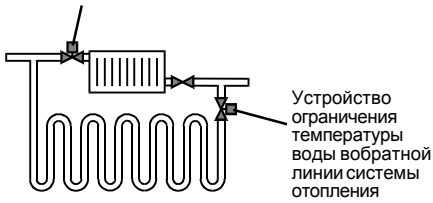
Вентиль термостата
