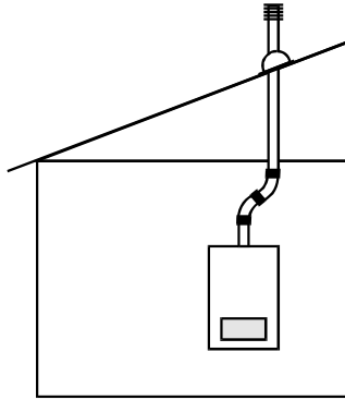
Вертикальная дымовая труба (с воздухопроводом и дымоходом "труба в трубе") ввод через наклонную кровлю С32х (см. стр. 15)
