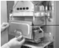
Крышка камеры сгорания
