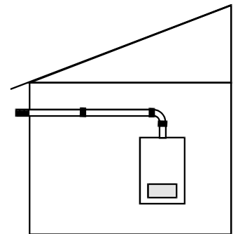
Горизонтальная дымовая труба (с воздухопроводом и дымоходом "труба в трубе") ввод через наружную стену С12х (см. стр. 16)
