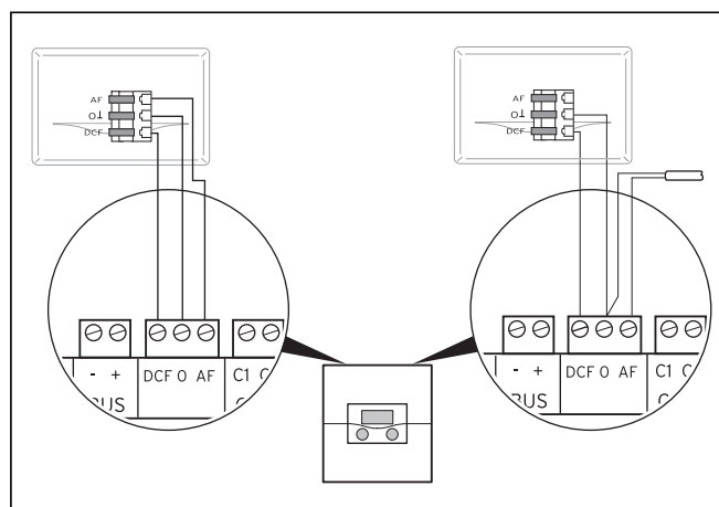
Рис. 5.11 Подключение DCF-приемника
