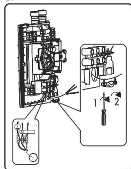
Рис.3 Монтаж ПЭВН Thermex Surf 5000, Surf 6000, Surf Plus 4500, Surf Plus 6000
