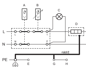
Рис. 5: Схема электрического подключения
