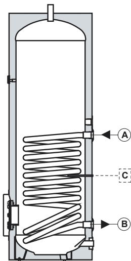
Места подключения водонагревателя VTI со стороны отопления.
