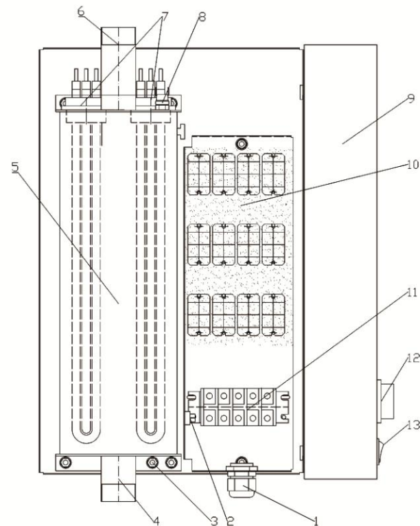
Рисунок 1. Устройство электродкотла. (крышка открыта)
