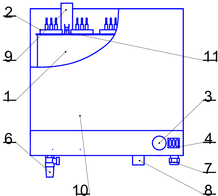
Рисунок 1. Схема электрокотла.
