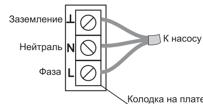
Рис.5 Подключение циркуляционного насоса
