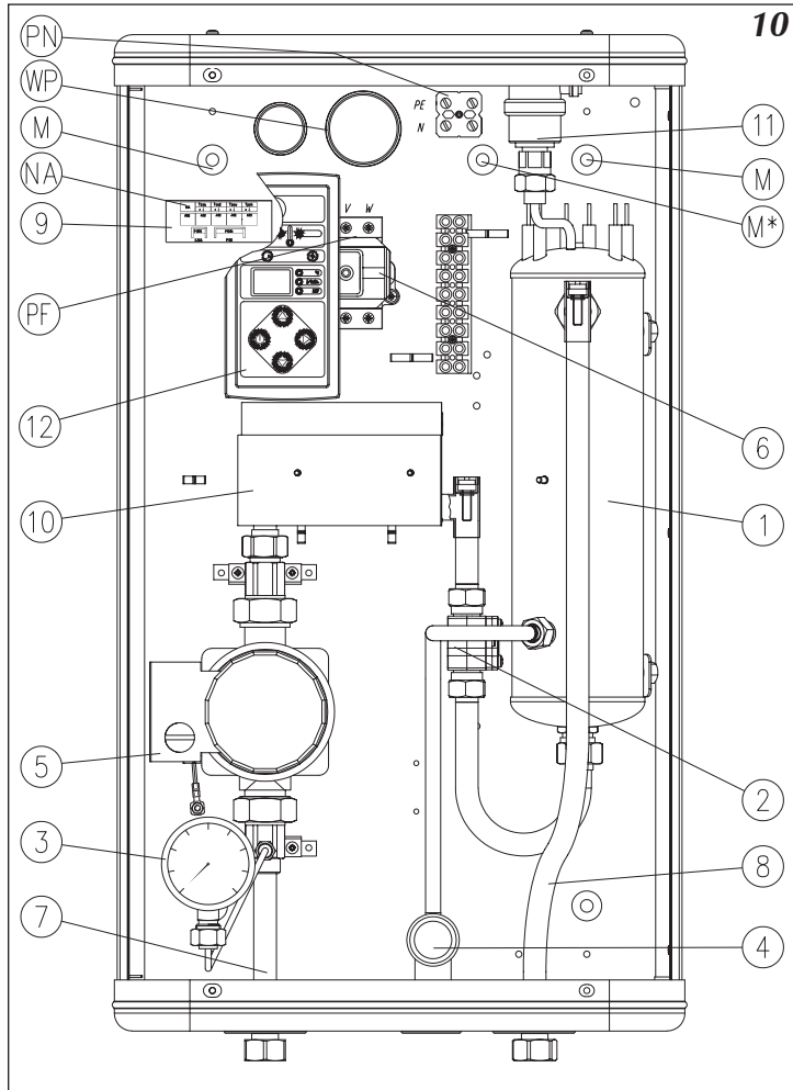
Рис. 10 Конструкция трехфазного котла ЕКСО.L
