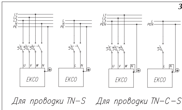
Рис.3 Подключение к электросети
