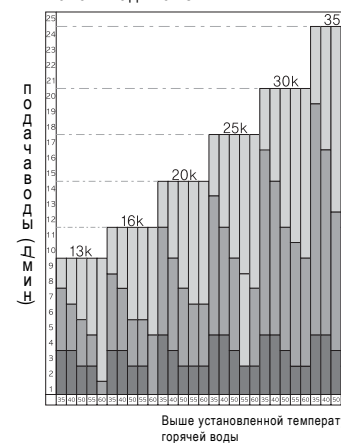
Температура поступающей в котел воды 5 °C.
