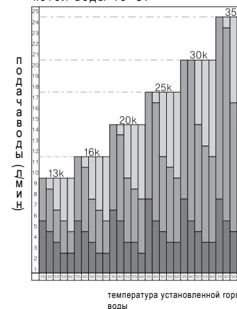
Температура поступающей в котел воды 15 °C.
