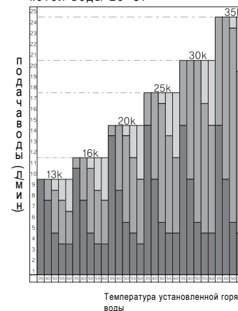
Температура поступающей в котел воды 25 °C.
