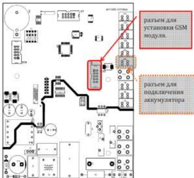
Рис 2. Вид платы управления котла
