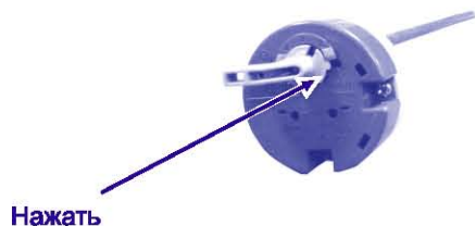
Рис.4. Расположение штока на термовыключателе термостата
