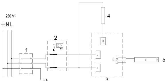
Рис. 5: Електрична схема
