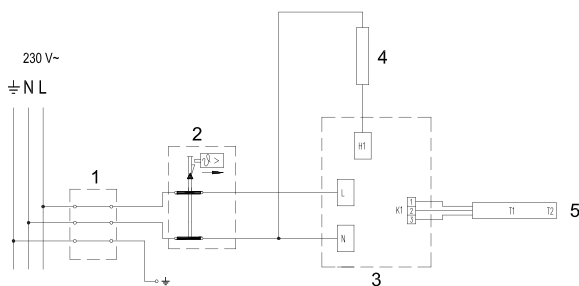
Fig. 5: Instalația electrică
