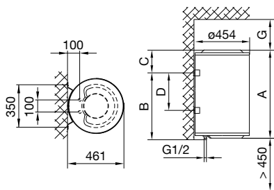
1 Сурет: Қабырғаға сатылас түрде жинақтау
