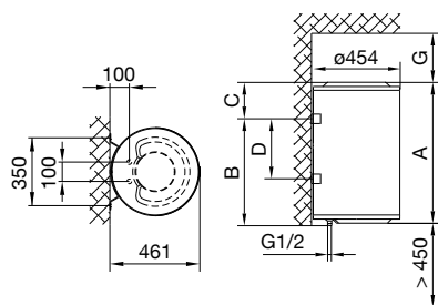
SI. 1: Vertikalno montiranje na zid
