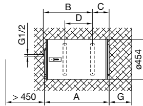
Мал. 2: Монтаж на стіну в горизонтальному положенні
