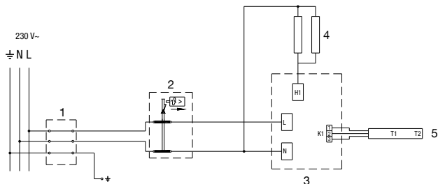
Мал. 6: Електросхема
