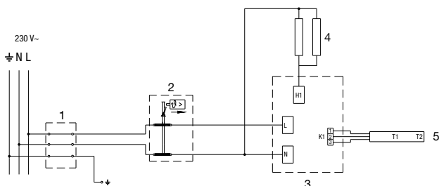
Fig. 6: Instalația electrică
