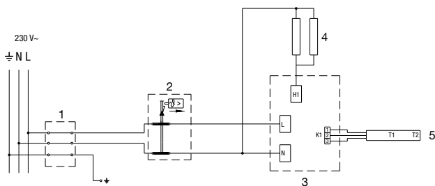
Рисунок 6: Электросхема
