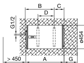
SI. 2: Horizontalno postavljanje na zid
