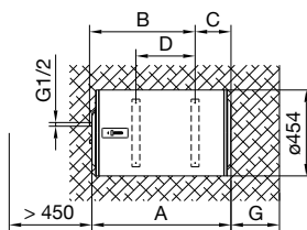
Fig. 2: Montare orizontală pe perete
