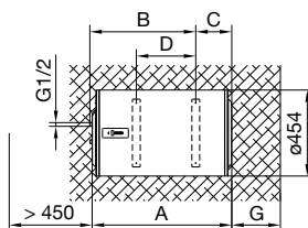
2 Сурет: Қабырғаға көлденен түрде жинақтау
