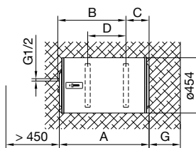
Рис. 2: Горизонтальный настенный монтаж
