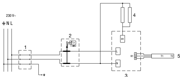
6 Сурет: Электр схемасы
