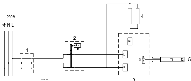
Sl. 6: Šema povezivanja električnih provodnika
