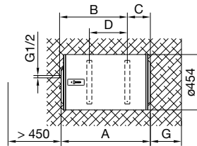
Мал. 2: Монтаж на стіну в горизонтальному положенні
