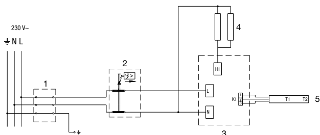
Fig. 6: Instalația electrică
