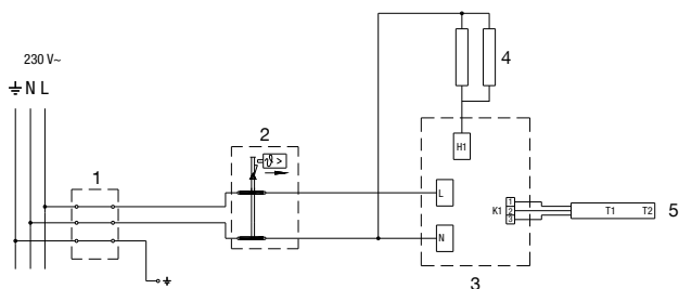
Fig. 6: Instalația electrică
