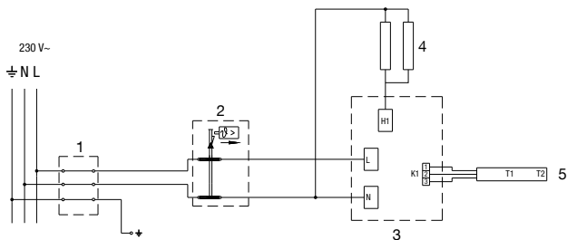
Рисунок 6: Электросхема
