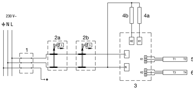
Fig. 6: Instalația electrică
