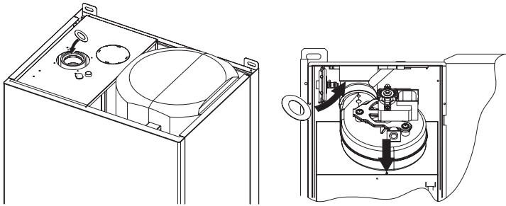
рис. 20 - Замена диафрагмы (А = если котел не установлен / В = Если котел и воздуховоды уже смонтированы)
