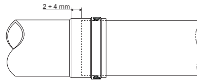
рис. 19 - Тепловое расширение
