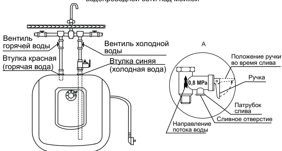
Схема подключения ЭВН к водопроводной сети под мойкой
