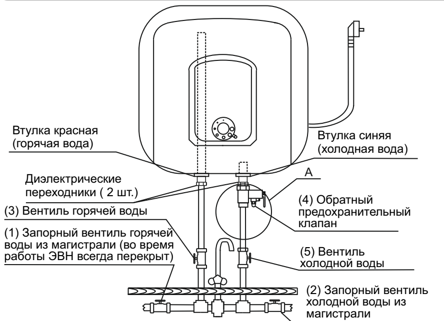
Схема подключения ЭВН к водопроводной сети над мойкой
