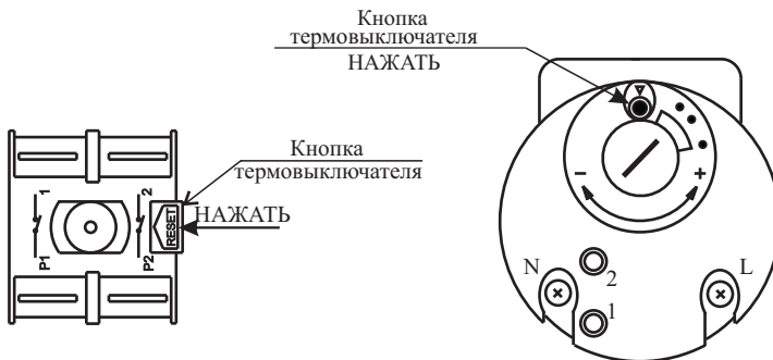
Рисунок 2 - Лицевые панели термовыключателей
