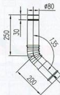
DGB-EL45 (Угол 45°)
