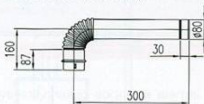
DGB-EL90 (Угол 90°)
