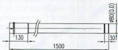
DGB-S1500 (Труба прямая 1500 мм.)
