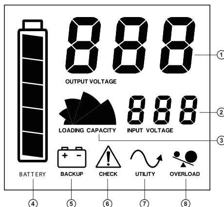
Рис. 1. LCD-дисплей ИБП
