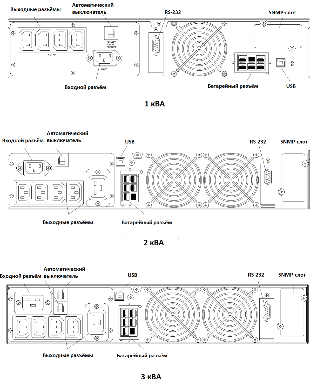
Рис.3. Задняя панель серии MRT (1-3 кВА)
