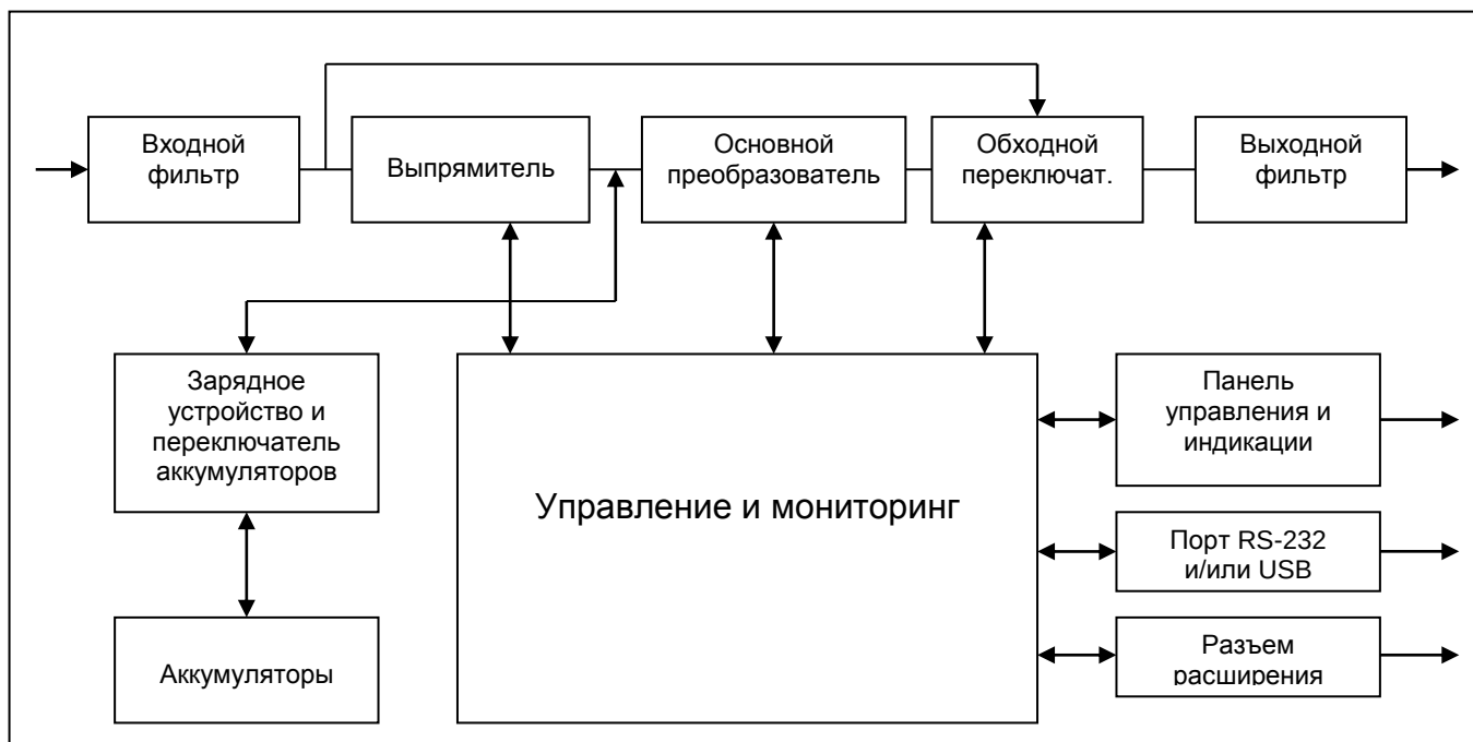
Рис. 7. Блок-схема ИБП
