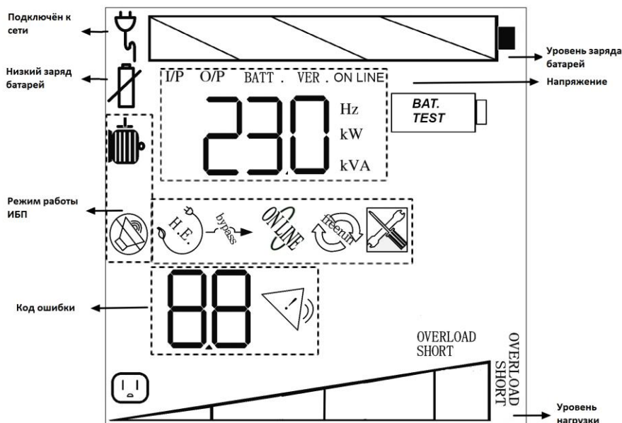
Рис. 8. ЖК-дисплей
