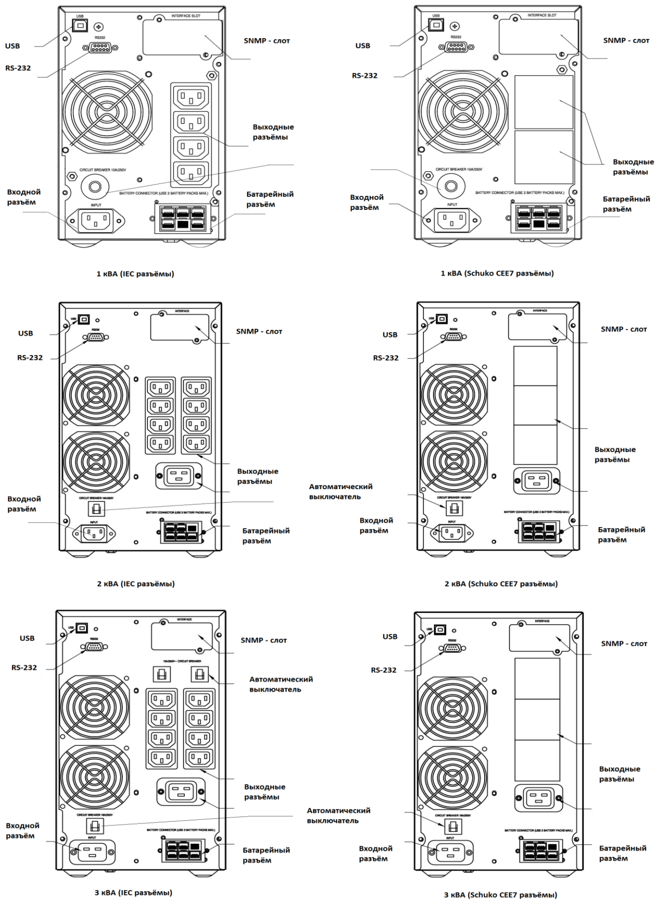
Рис. 4. Задняя панель серии MAC
