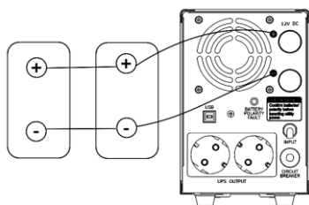
Fig. 3 12V DC
