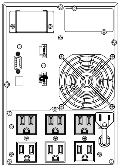
Рисунок 45. Модель PW9130L1500T-XL
