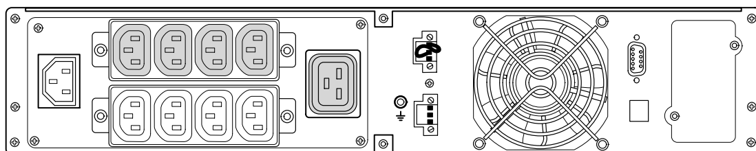
Рисунок 37. Модели PW9130i2000R-XL2U, PW9130G2000R-XL2UEU
