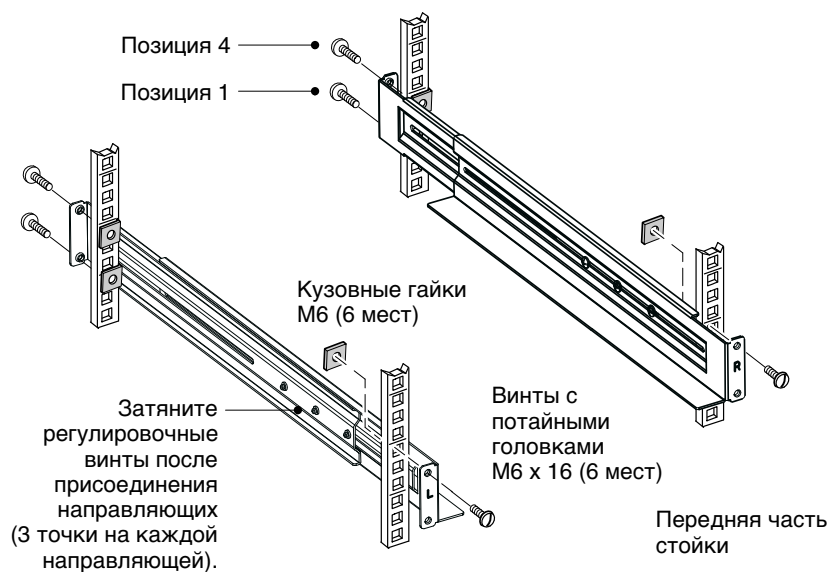
Рисунок 5. Крепление направляющих
