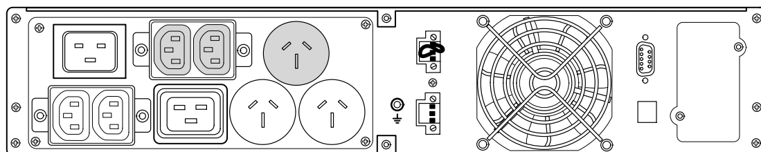
Рисунок 42. Модель PW9130G3000R-XL2UAU
