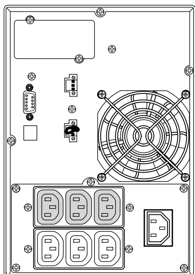
Рисунок 51. Модель PW9130i700T-XL
