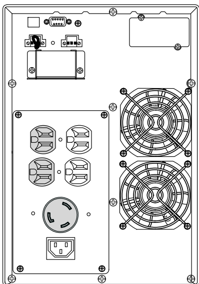
Рисунок 49. Модель PW9130G2000T-XL
