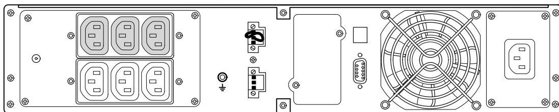
Рисунок 34. Модель PW9130i1500R-XL2U
