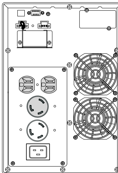
Рисунок 50. Модель PW9130G3000T-XL
