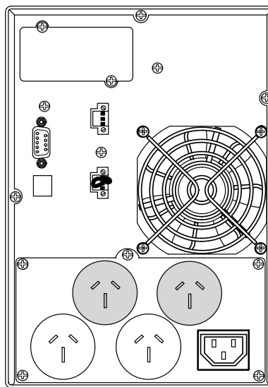
Рисунок 56. Модель PW9130G700T-XLAU
