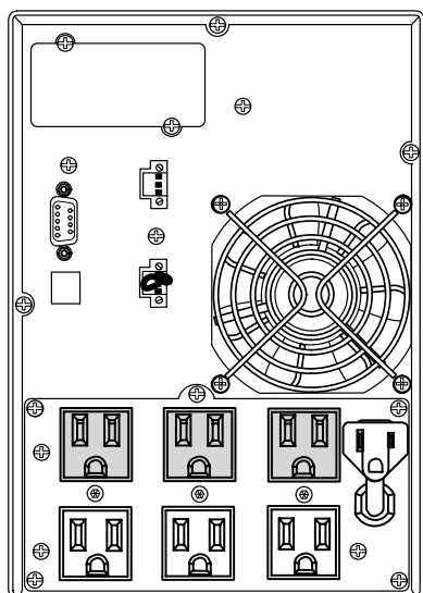
Рисунок 43. Модель PW9130L700T-XL
