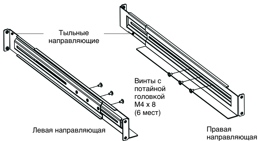
Рисунок 4. Сборка направляющих
