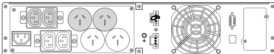
Рисунок 38. Модель PW9130G2000R-XL2UAU
