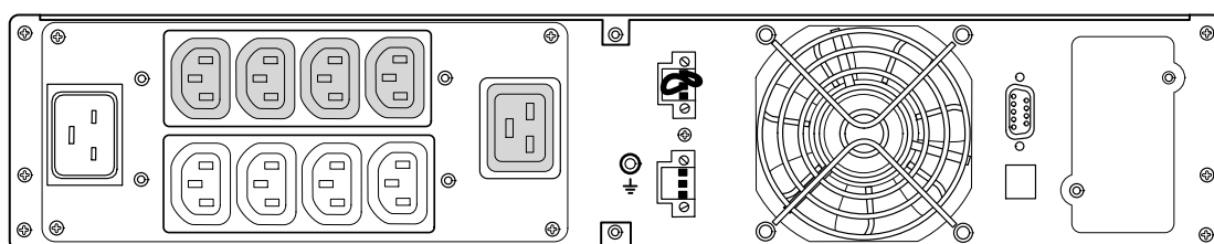
Рисунок 41. Модели PW9130G2500R-XL2UEU, PW9130i3000R-XL2U, PW9130G3000R-XL2UEU
