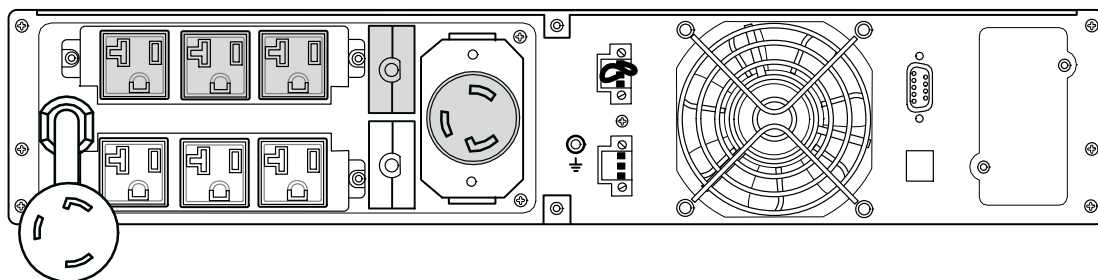
Рисунок 39. Модели PW9130L2500R-XL2U, PW9130L3000R-XL2U
