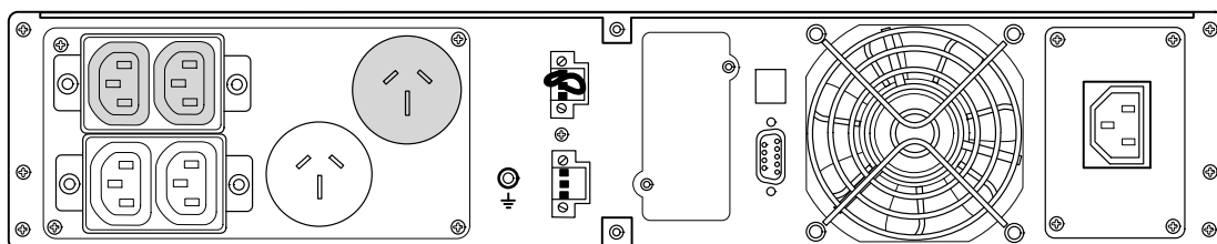
Рисунок 32. Модель PW9130G1500R-XL2UAU
