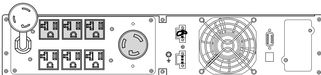
Рисунок 35. Модель PW9130L2000R-XL2U
