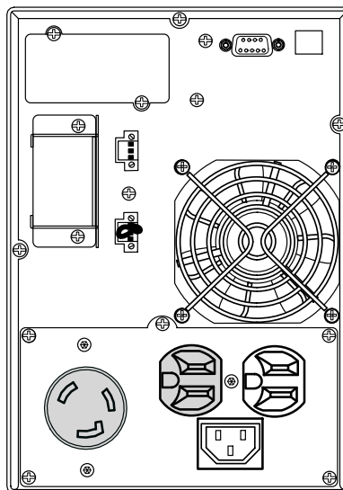
Рисунок 48. Модель PW9130G1000T-XL
