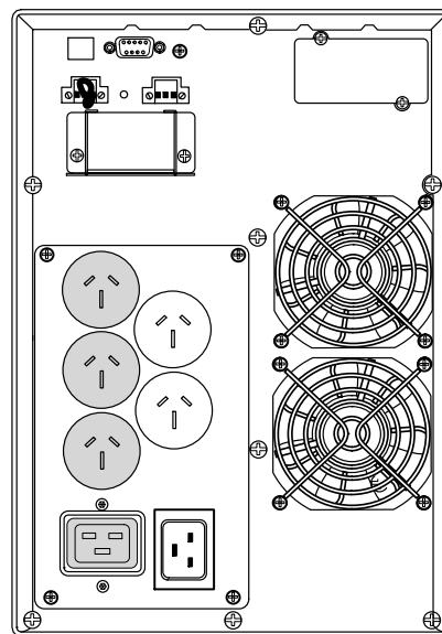
Рисунок 60. Модель PW9130G3000T-XLAU
