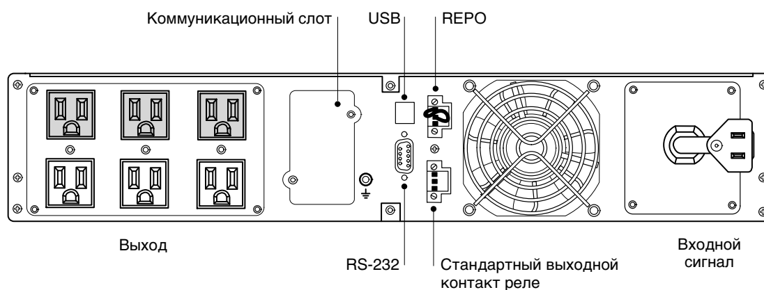
Рисунок 18. Коммуникационные устройства и клеммы управления (показана модель PW9130L1000R-XL2U)
