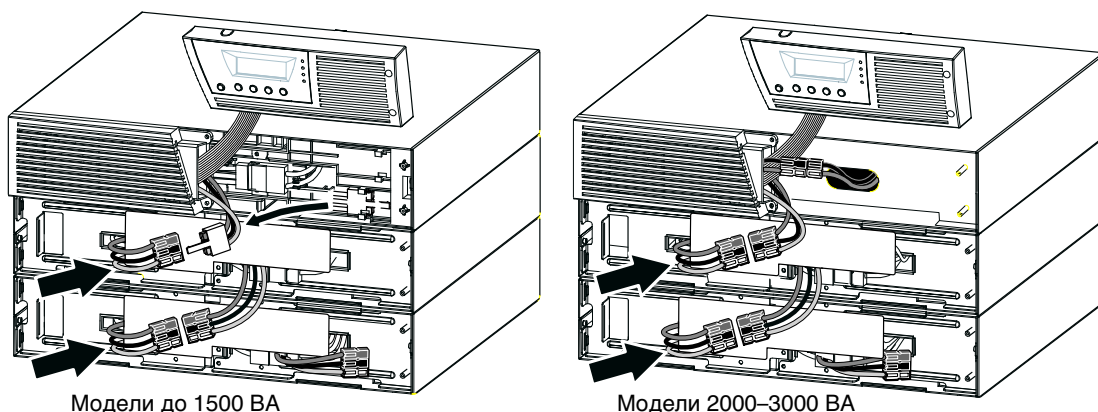
Рисунок 13. Типичная ЕВМ установка
