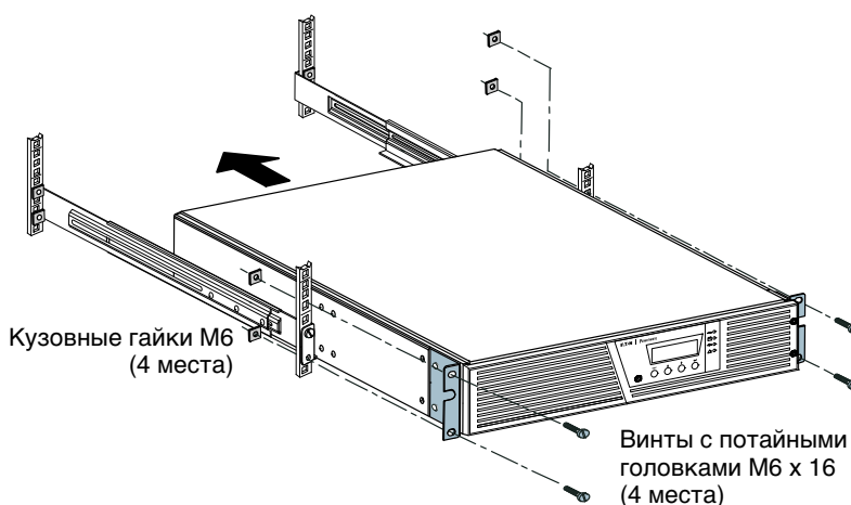
Рисунок 7. Крепление передней части корпуса
