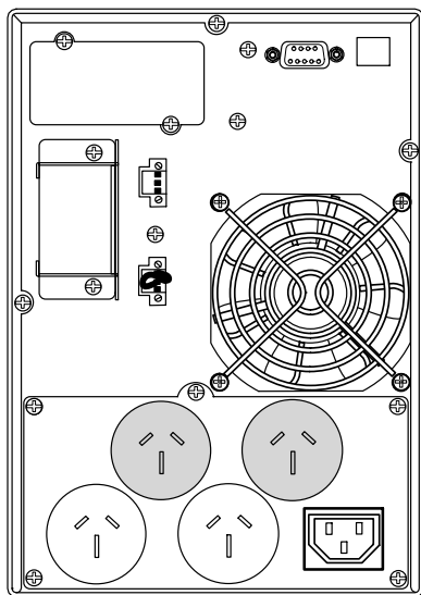
Рисунок 57. Модель PW9130G1000T-XLAU
