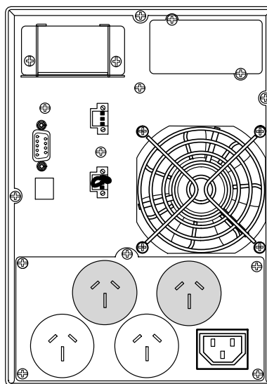
Рисунок 58. Модель PW9130G1500T-XLAU
