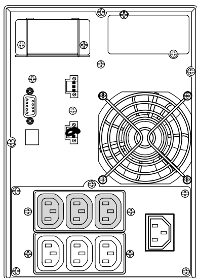
Рисунок 53. Модель PW9130i1500T-XL
