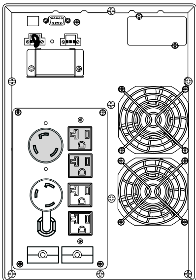
Рисунок 47. Модель PW9130L3000T-XL
