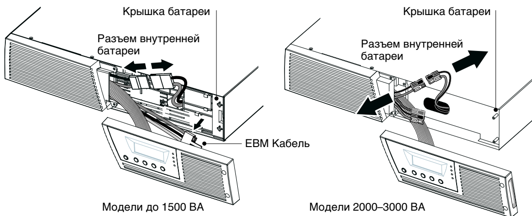
Рисунок 24. Отключение внутренних батарей ИБП (показано без EBM)
