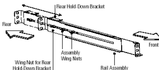
Рисунок 3. Регулировка глубины рейки
