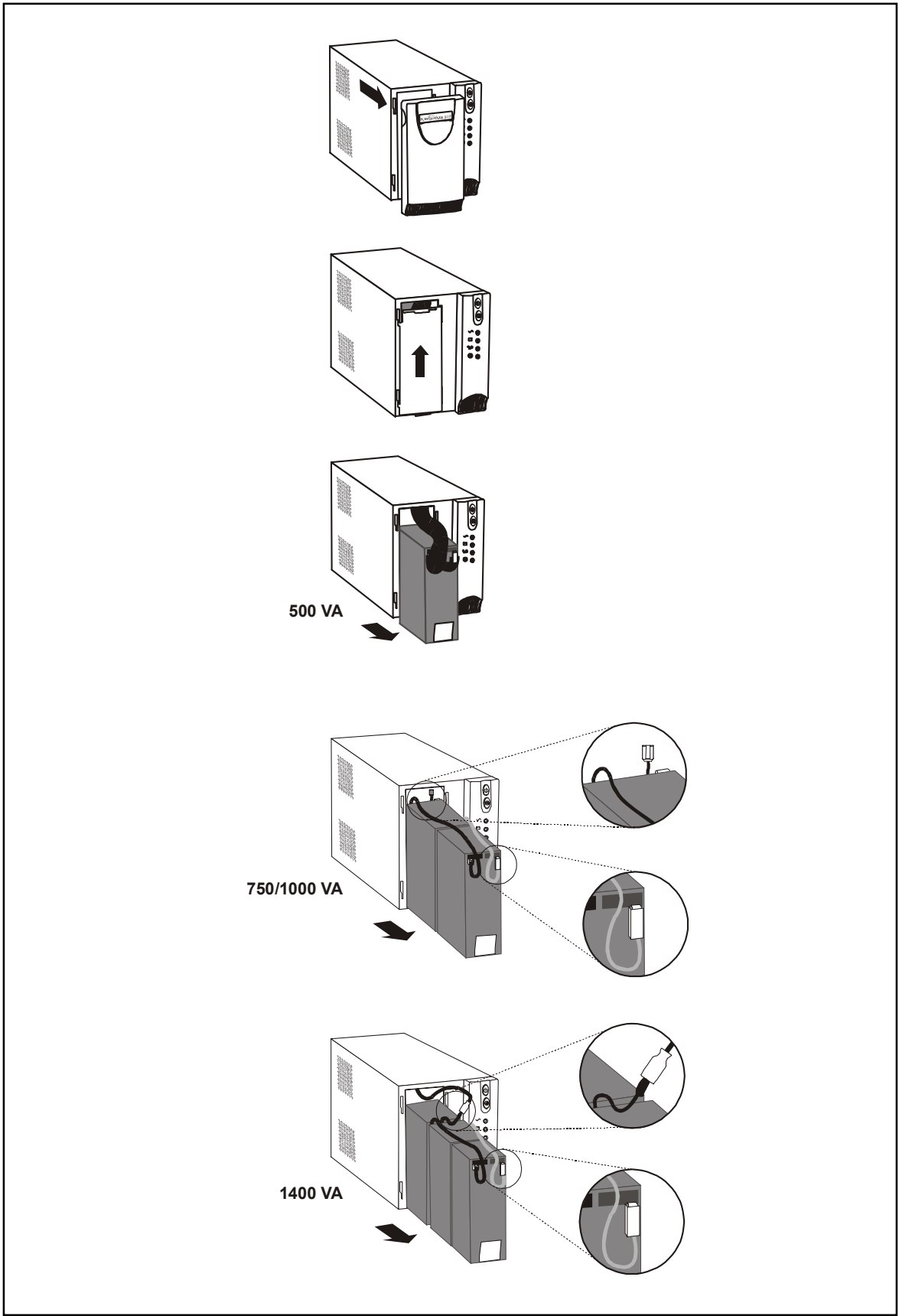
Рисунок 9. Замена батарей
