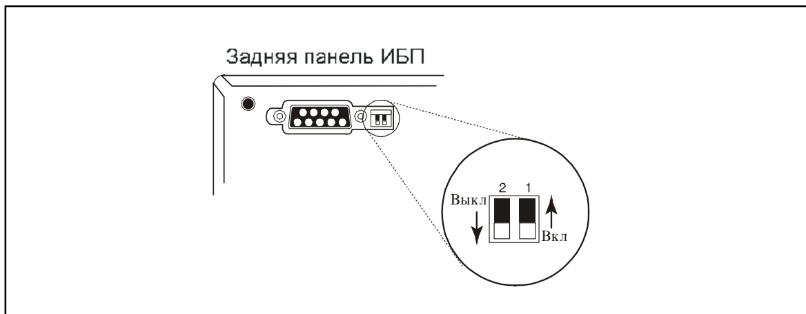
Рисунок 5. DIP переключатели
