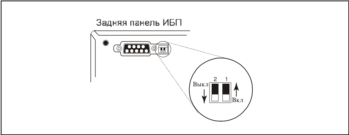
Рисунок 5. DIP переключатели
