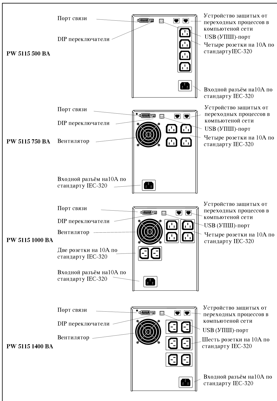
Рисунок 3. Задние панели
