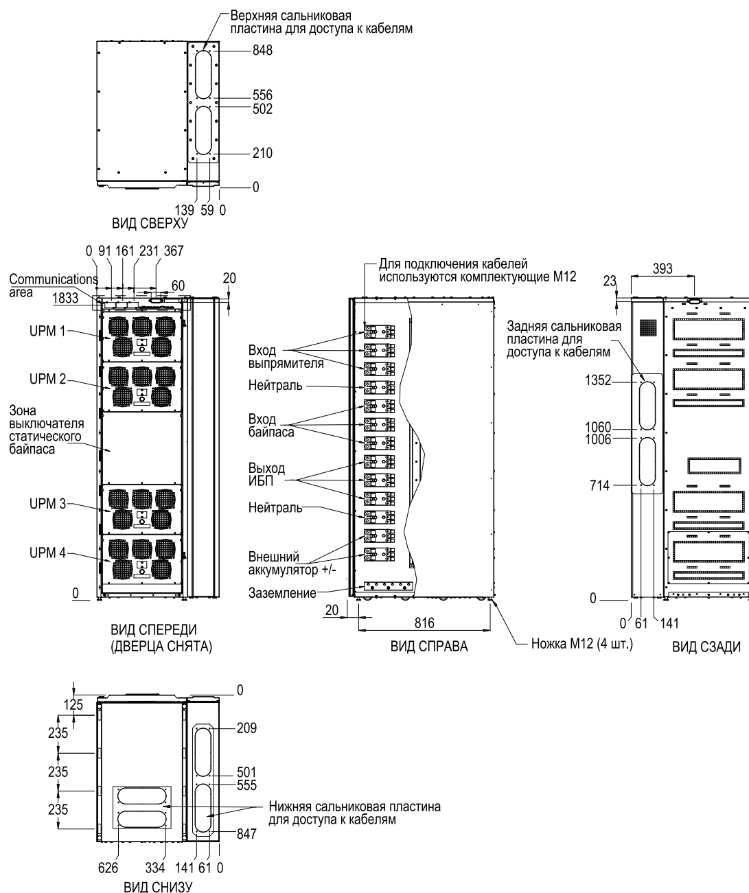
Рис. 4-3: Расположение сальниковых панелей и разъемов в ИБП 93PM 160-200 кВт
