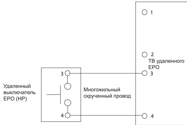
Рис. 4-15: Проводка нормально-разомкнутого удаленного выключателя EPO
