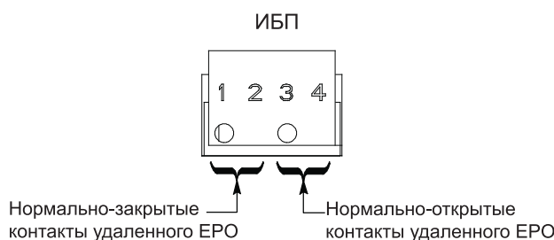
Рис. 4-14: Назначение разъемов клеммного блока удаленного выключателя ЕРО
