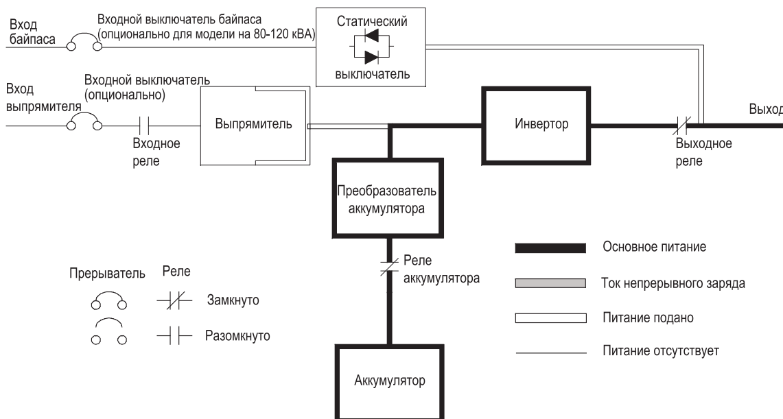
Рис. 5-4: Путь прохождения тока через ИБП в режиме работы от аккумулятора
