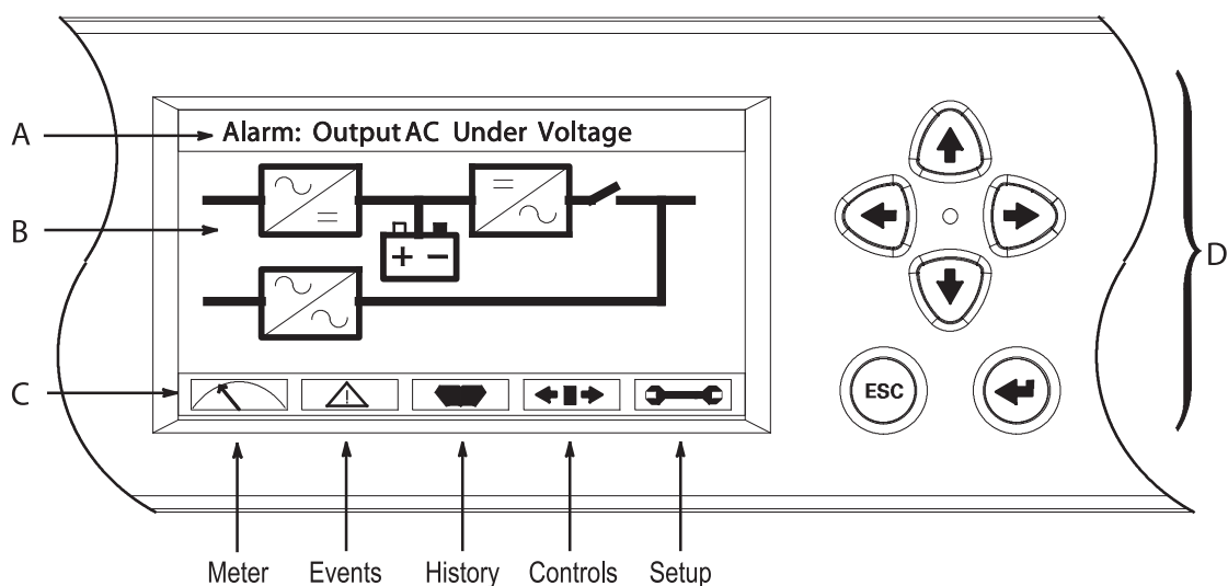
Рис. 6-4: Элементы ЖК-экрана
