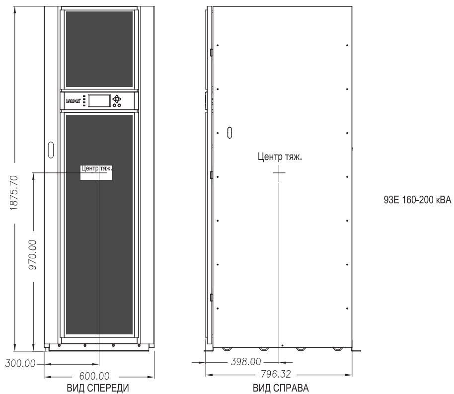
Рис. 3-3: Центр тяжести шкафа ИБП
