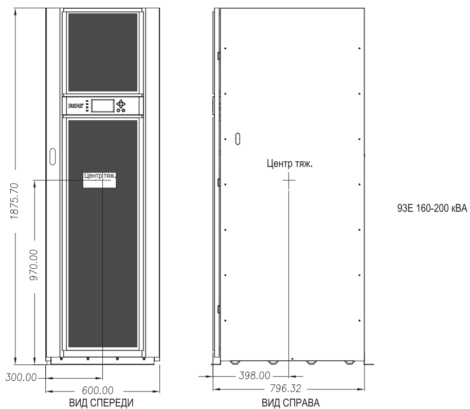
Рис. 3-3: Центр тяжести шкафа ИБП
