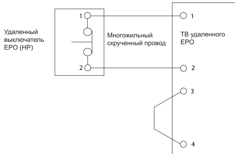
Рис. 4-16: Проводка нормально-замкнутого удаленного выключателя EPO
