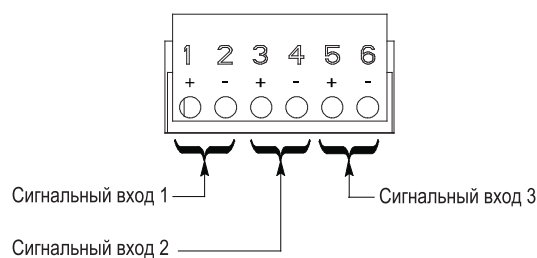
Рис. 4-9: Расположение разъемов в клеммной коробке сигнального входа
