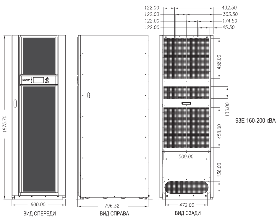
Рис. 3-1: Габариты шкафа ИБП (виды спереди и справа)
