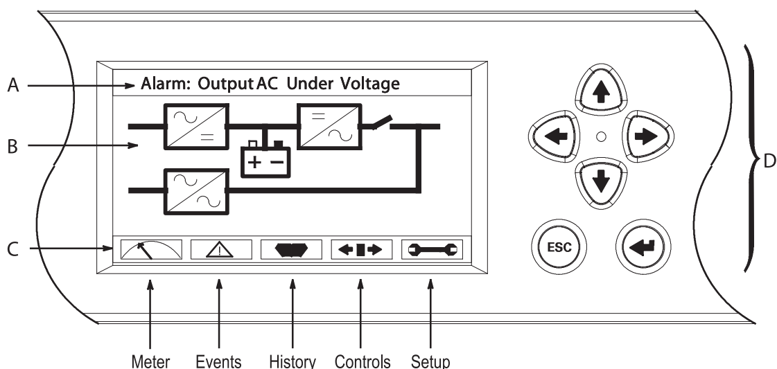
Рис. 6-4: Элементы ЖК-экрана
