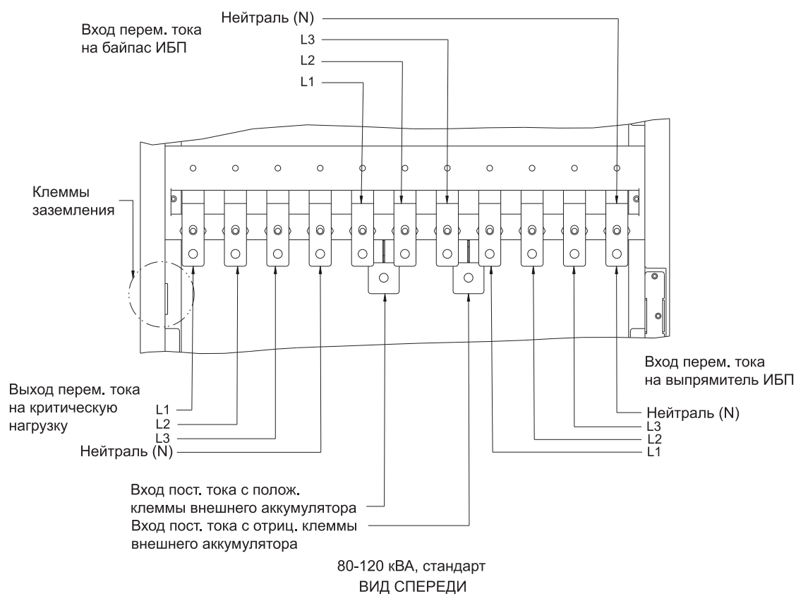
Рис. 4-5: Расположение узлов клемм 80-120 кВА
