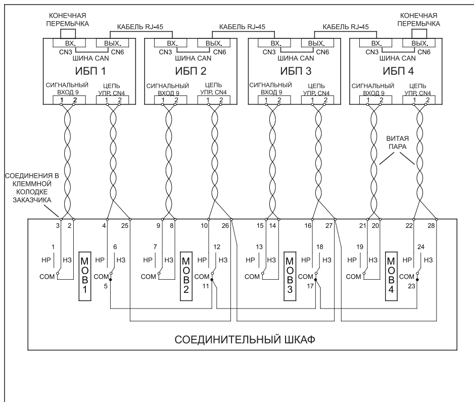
Рис. 4-12: Управляющая проводка параллельного ИБП
