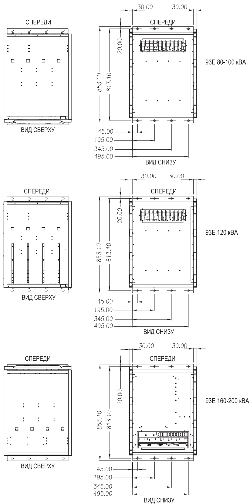
Рис. 3-2: Габариты шкафа ИБП (виды сверху и снизу)
