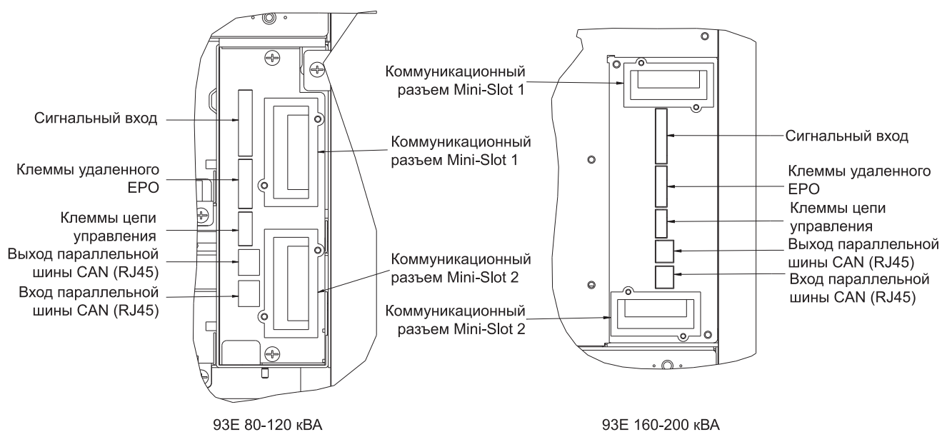
Рис. 4-7: Расположение интерфейсных клемм
