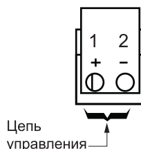
Рис. 4-11: Назначение разъемов клеммного блока управляющей цепи
