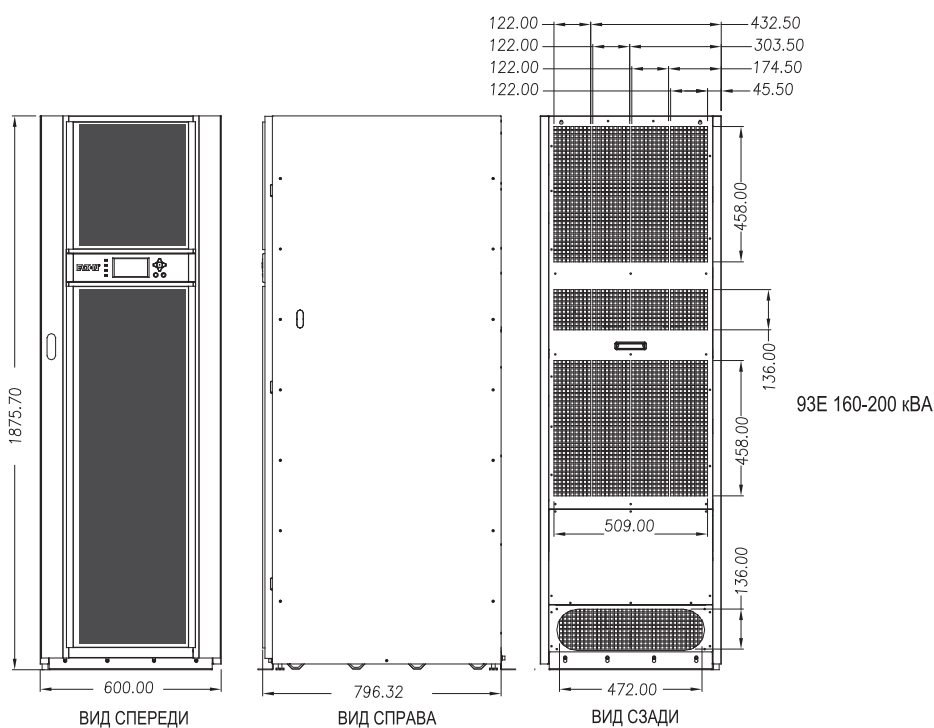
Рис. 3-1: Габариты шкафа ИБП (виды спереди и справа)
