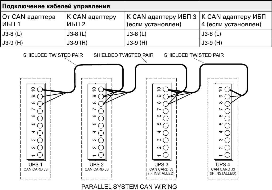
Рисунок 45. Монтаж информационных кабелей
