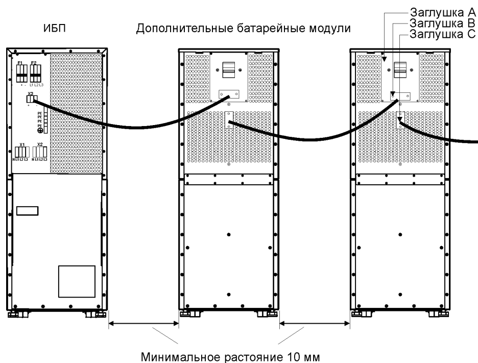
Рисунок 18. Схема соединения ИБП и батарейных модулей
