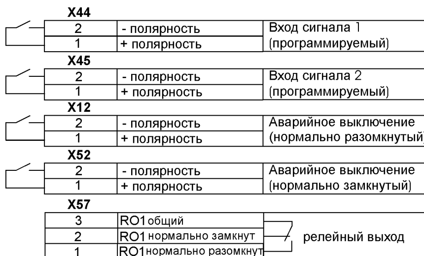
Рисунок 22. Подключение к ИБП кабелей внешних управляющих устройств
