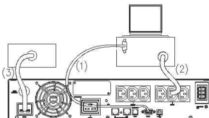
Рис. 3-4.2. Подключение ИБП на 2 и 3 кВА
