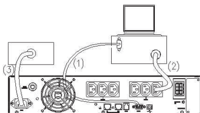
Рис. 3-4.1. Подключение ИБП на 1 кВА
