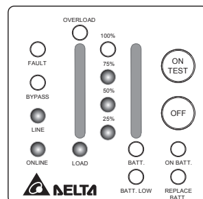
Рис. 3-6. Индикация в режиме двойного преобразования
