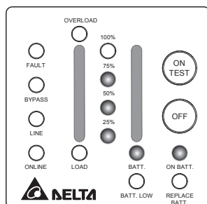
Рис. 3-7. Индикация в режиме питания от батарей
