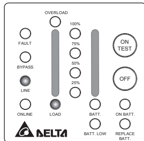
Рис. 3-5 Индикация в режиме ожидания
