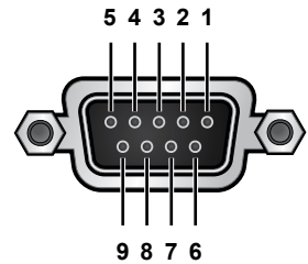
Рис. 3-7. Порт RS-232
