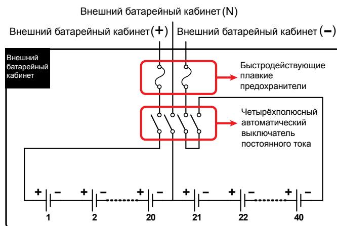
Рис. 5-15. Подключение внешнего батарейного шкафа
