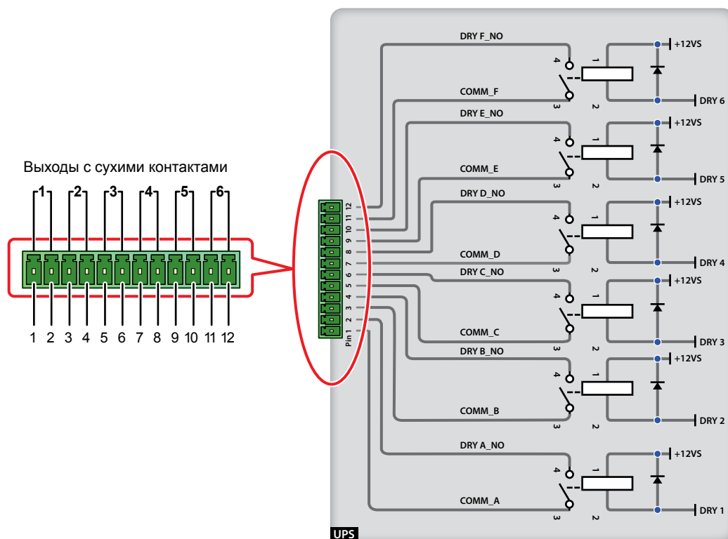
Рис. 3-11: Выходы с сухими контактами
