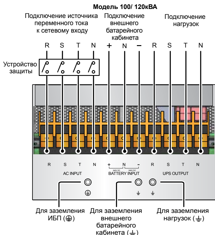
Рис. 5-7. ИБП DPS 100/ 120кВА. Схема установки устройств защиты
