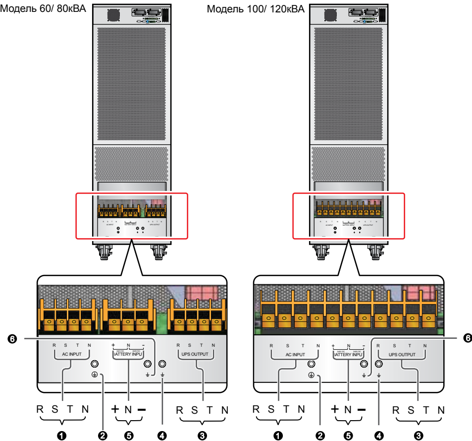
Рис. 5-9. Блок выводов ИБП
