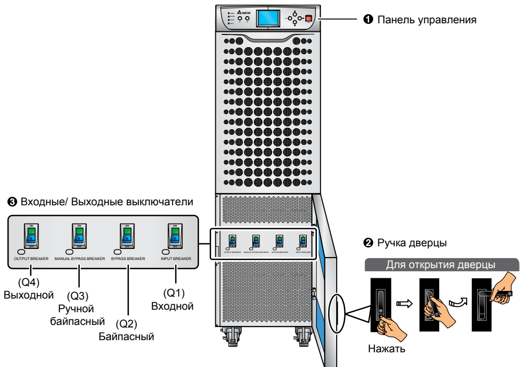
Рис. 3-3. Вид спереди
