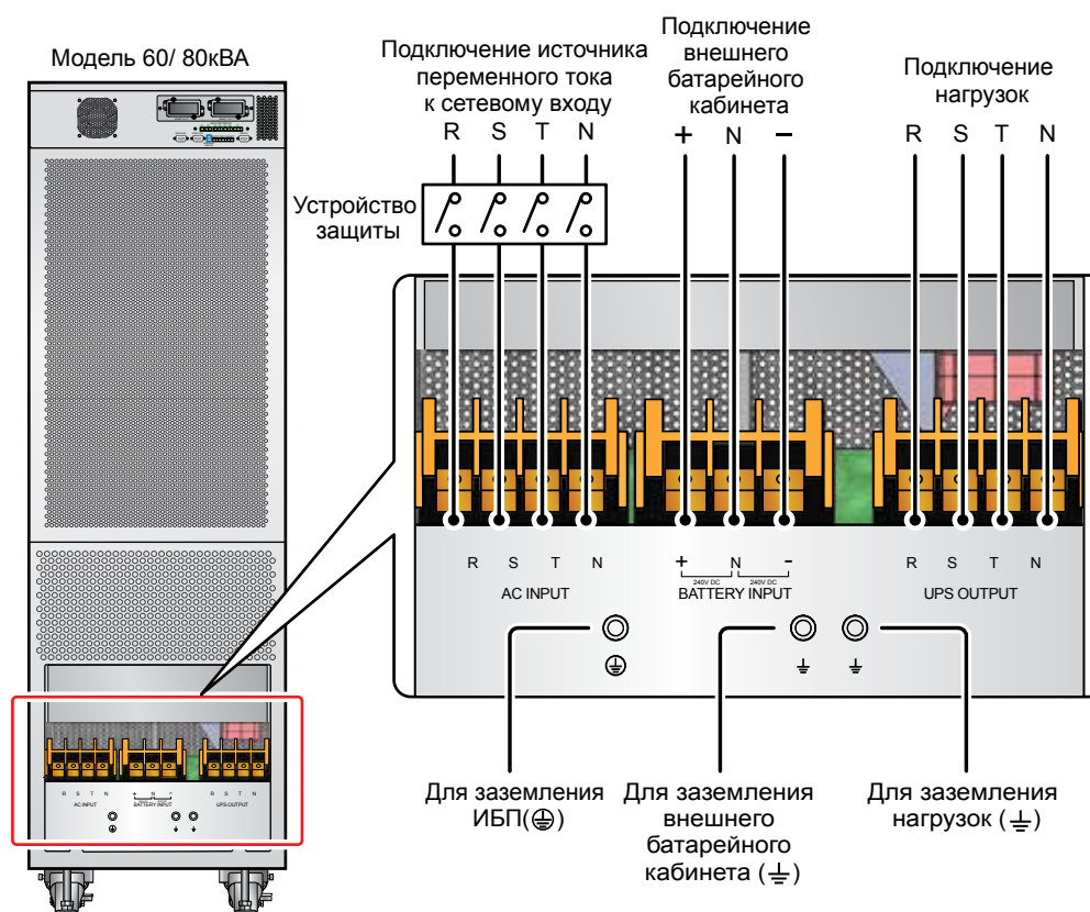
Рис. 5-10. Подключение ИБП DPS 60/ 80 кВА
