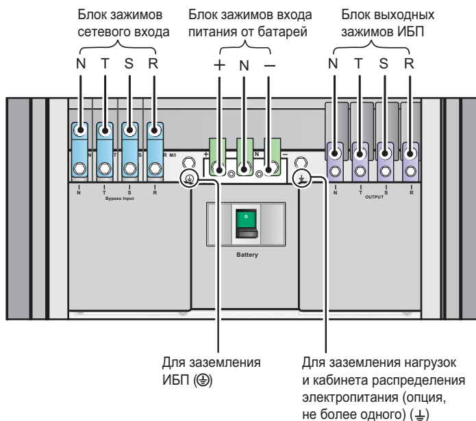
Рис. 5-7. Схема подключения в конфигурации с одним входом (одиночный ИБП)
