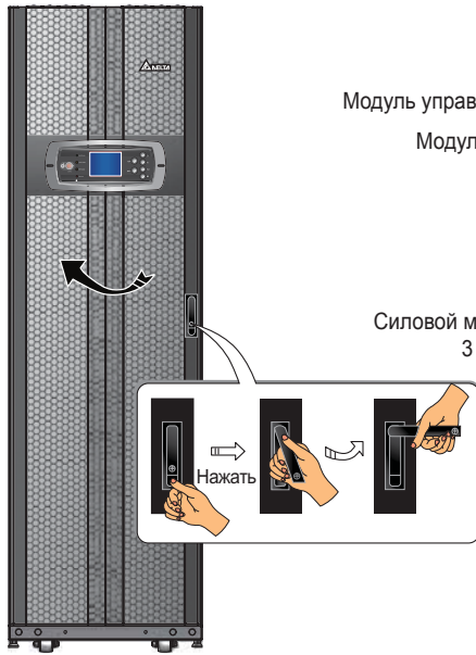
Рис. 2-4. Вид спереди
