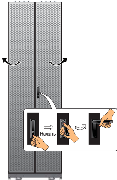
Рис. 2-6. Вид сзади
