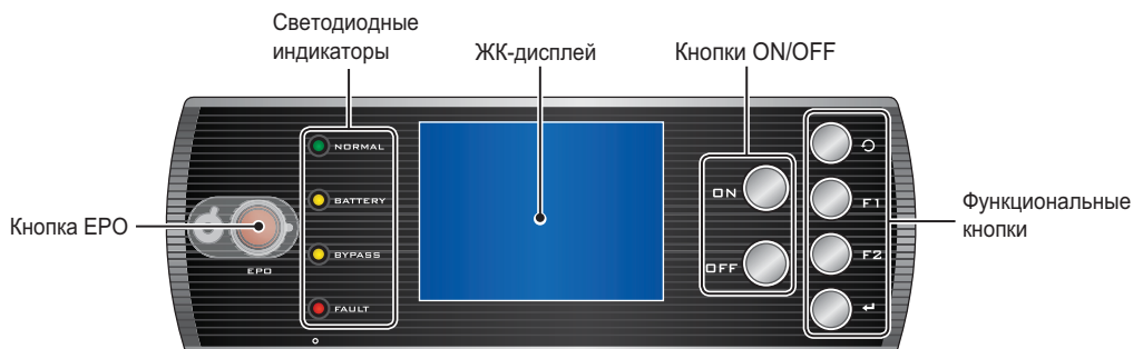
Рис. 7-2. Панель управления
