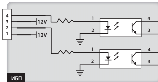
Рис. 4-6. Входы с сухими контактами (два комплекта)
