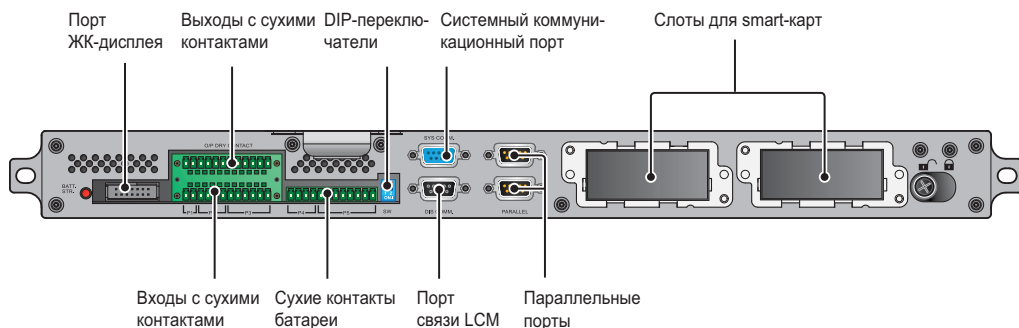
Рис. 4-2. Коммуникационные интерфейсы
