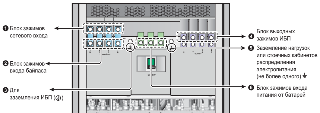
Рис. 5-5. Выводы ИБП
