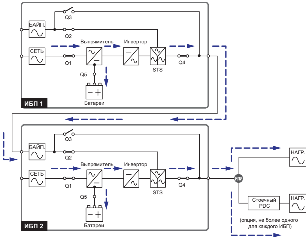
Рис. 3-10. Последовательное резервирование
