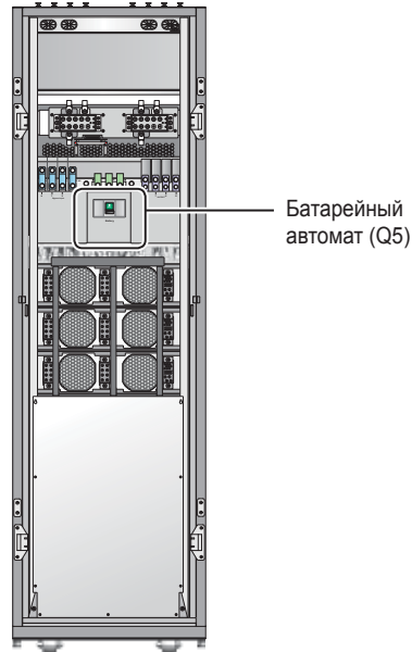
Рис. 2-7 Вид сзади с открытой дверцей
