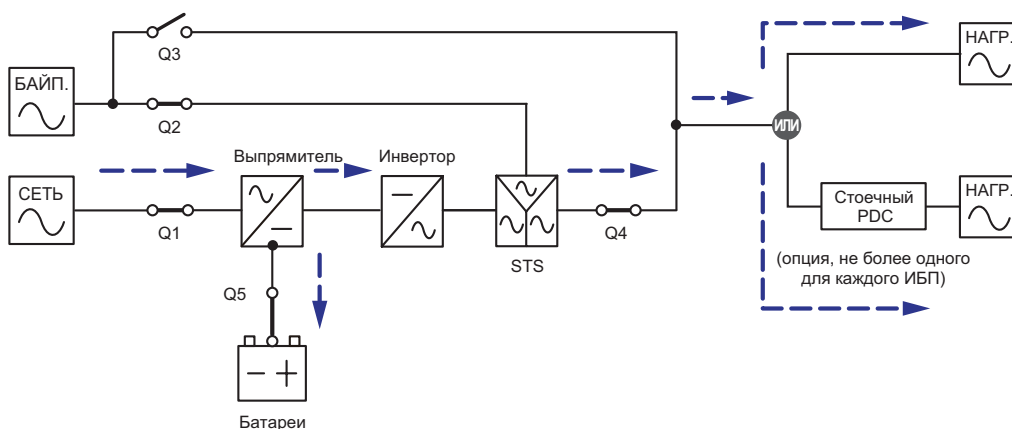
Рис. 3-1. Нормальный режим работы, система с одним ИБП
