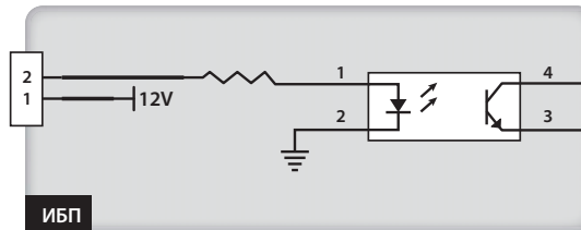
Рис. 4-5. Сухие контакты батареи
