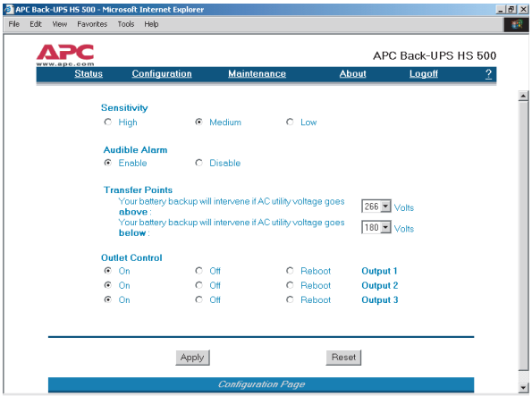
Рисунок 16. Окно настройки
