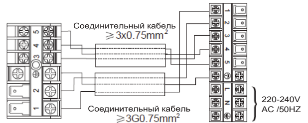
Внутренний блок Наружный блок
