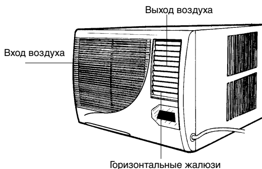
Установка и устройство оконного кондиционера
