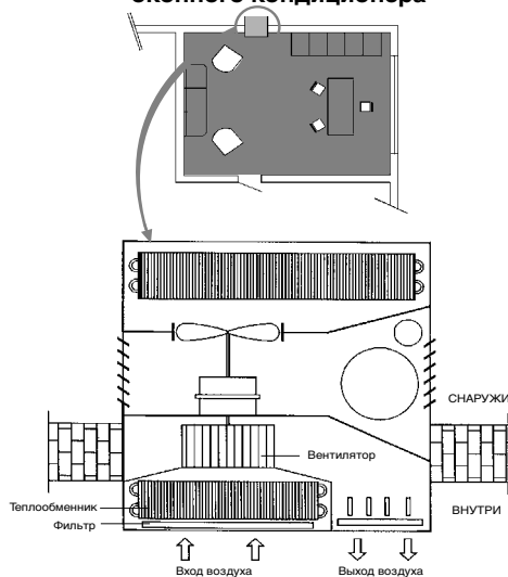
Установка и устройство оконного кондиционера
