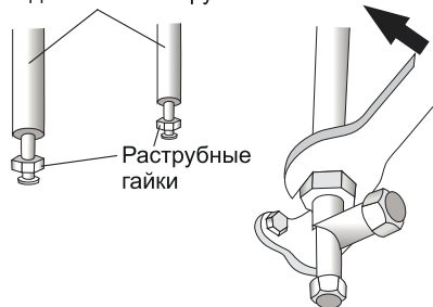
Соединительные трубы
